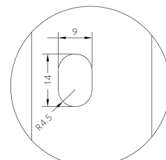
I部取付固定穴拡大図
